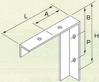
1.L型ブラケット
