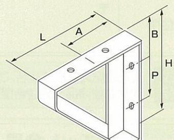
3.三角ブラケット 補強=アングル
