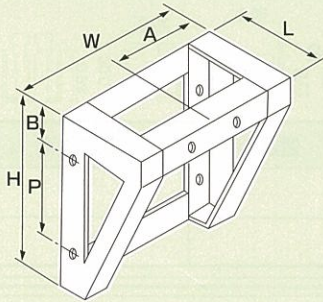
4.三角ブロック型ブラケット
