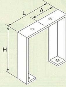
5.門型ブラケット ベース付
